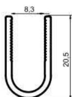
K-1111 128 gr/m
