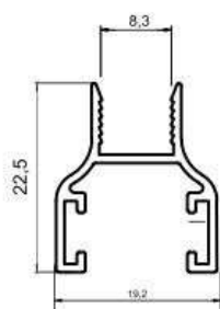
K-1086 200 gr/m
