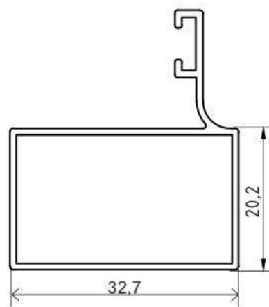
K-1061 320 gr/m
