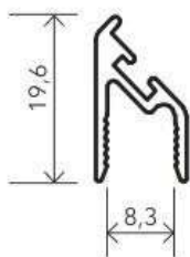
K-1100 164 gr/m
