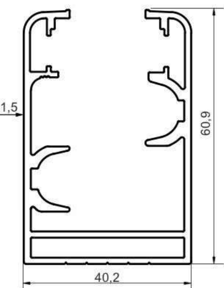
K-1033 1222 gr/m
