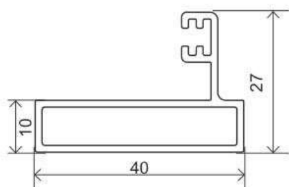
K-1051 457 gr/m
