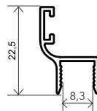
K-1096 139 gr/m
