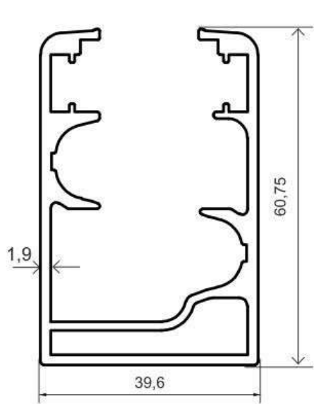
K-1030 1377 gr/m
