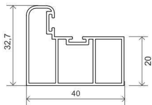
K-1220 515 gr/m
