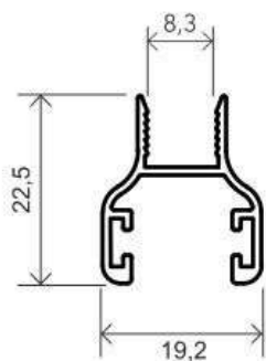
K-1085 207 gr/m
