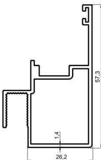
K-1150 651 gr/m
