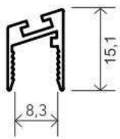
K-1105 131 gr/m
