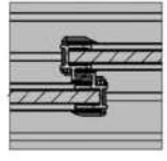
DETAY E ÖLÇEK 2 : 5
